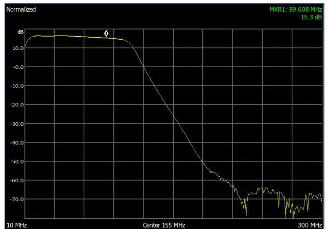
周波数-利得(10MHz-300MHz)
