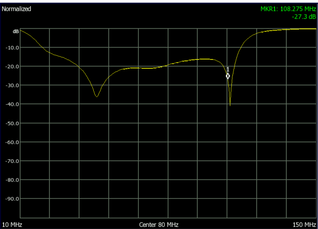
OUT Returnloss (10-150MHz)
