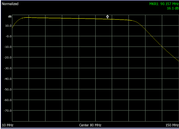
周波数-利得(10MHz-150MHz)
