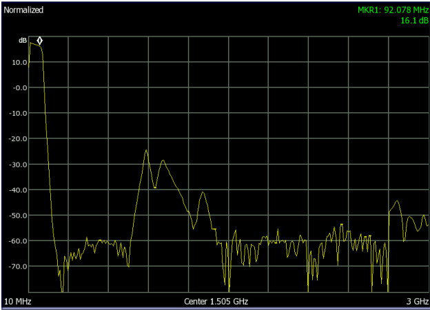
周波数-利得(10MHz-3000MHz)
