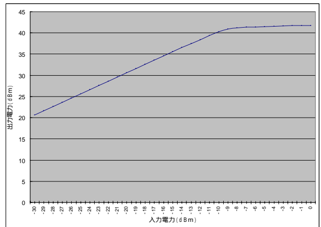
入出力特性(@83.0MHz ) @24
