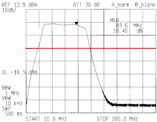
周波数 - 利得(@-15dBm入力) @24
